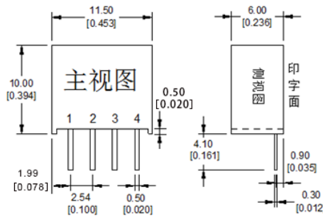
封装尺寸图
